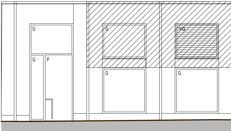
FASAD MOT GÄRDEN
